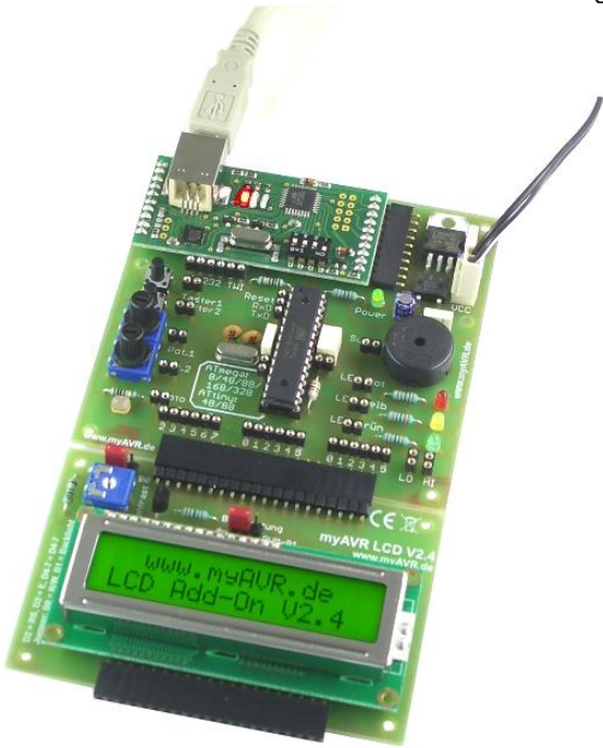
Abbildung / picture: myAVR Board MK2 mit myAVR LCD Add-On myAVR board MK2 with myAVR LCD Add-On
